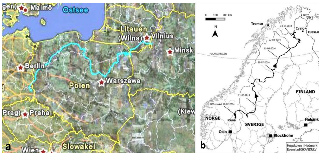
Figure 2 Exemples de distances parcourues par le loup en phase de dispersion* (suivi GPS/GSM) ; a) distance équivalente à 800 km en ligne droite en Allemagne entre le 23/04 et le 12/10/2009 (I. Reinhardt, Lupus Consulting). b) distance équivalente à 1200 km en ligne droite en Suède entre le 12/02 et le 24/10/2014 (C. Milleret, Skandulv).
